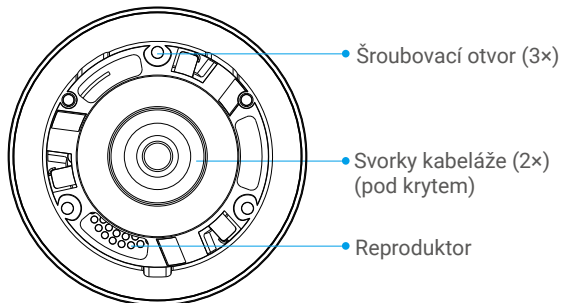
Spodní pohled
